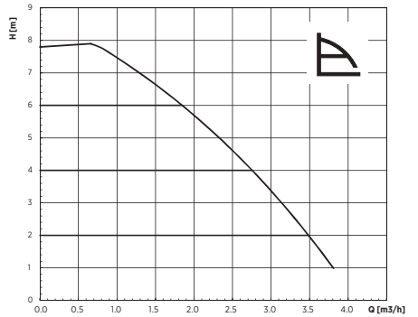
Sabit Basiñç
