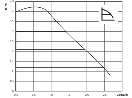
Sabit Basiñç
