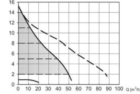
D65-150 F
