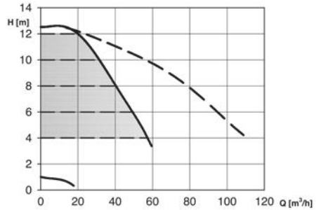
D80-120 F
