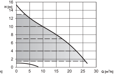
40-150 F
