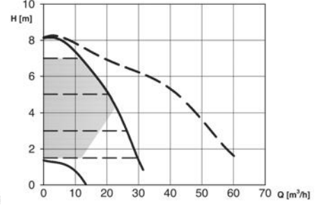
D65-80 F
