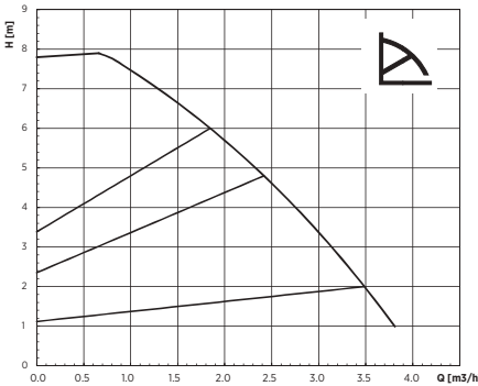
Oransal Basiñç
