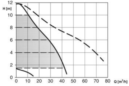
D65-120 F
