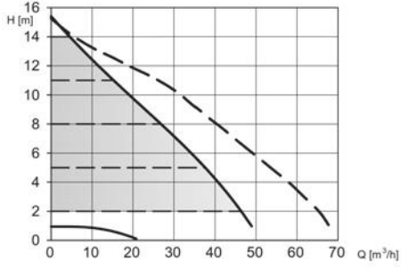
D50-150 F
